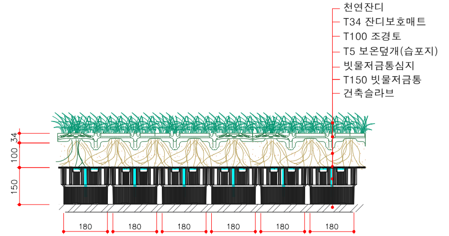
7 빗물저금통 '옥상녹화' 설치도 SCALE : NONE
