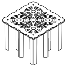
5 이동지지판 등각도 SCALE = NONE
