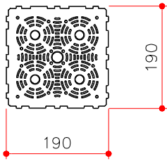
3 이동지지판 평면도 SCALE = NONE
