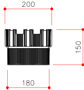
2 빗물저금통 정면도 SCALE = NONE
