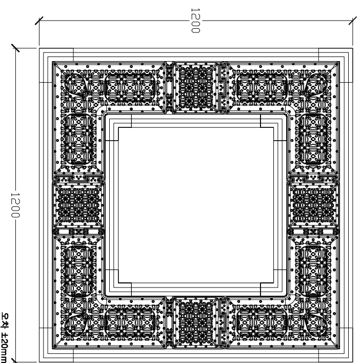
1 가로수보호판 및 보호틀 SCALE : NONE
