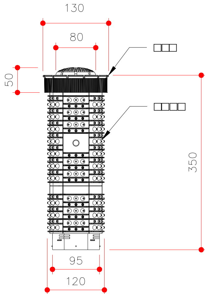
4 생육삼통관 정면도 SCALE = NONE
