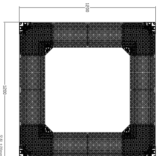
1 가로수보호판 및 보호틀 SCALE : NONE 오차 ±20mm
