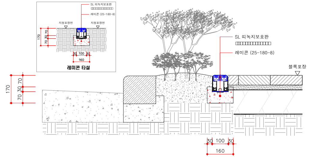
6 2-2' 레미콘타설 설치도 SCALE : NONE
