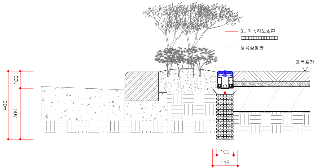
5 1-1' 생육상통관 결합 설치도 SCALE : NONE
