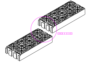
4 보호판 체결 상세도 SCALE = NONE
