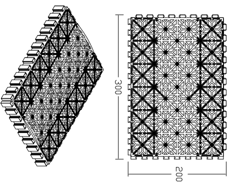
5. 가로수 보호판 A형
