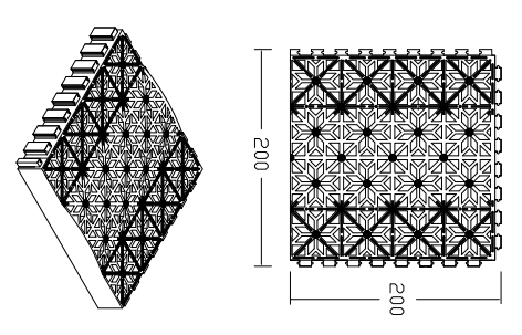
6. 가로수 보호판 B형
