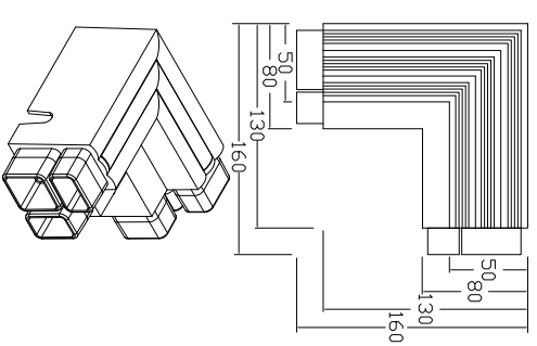
3. 외측 사각 소켓
