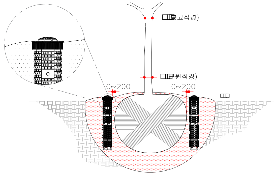
5 생육삼통관 설치도 SCALE = NONE
