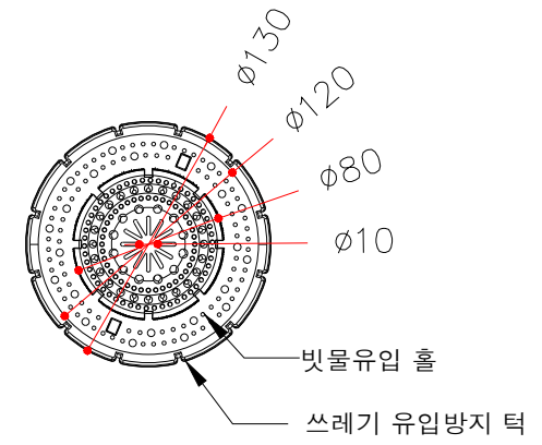
3 생육삼통관 CAP 평면도 SCALE = NONE
