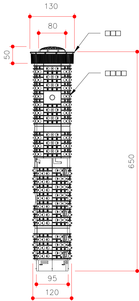
4 생육삼통관 정면도 SCALE = NONE
