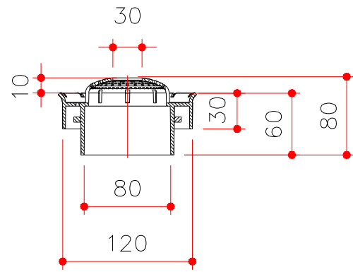
1 생육삼통관 CAP 단면도 SCALE = NONE
