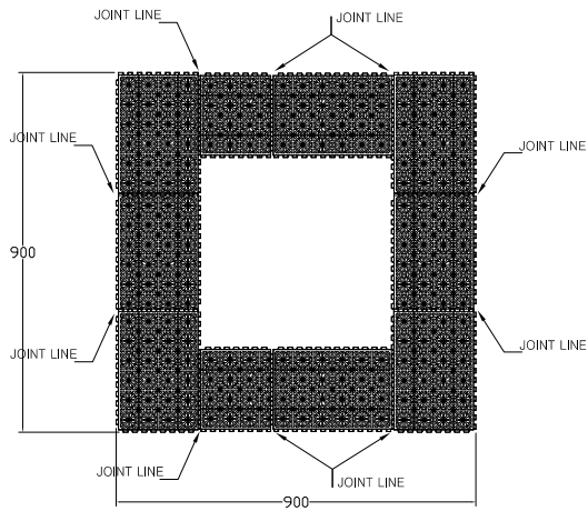
3 보호판 상세도 SCALE : NONE
