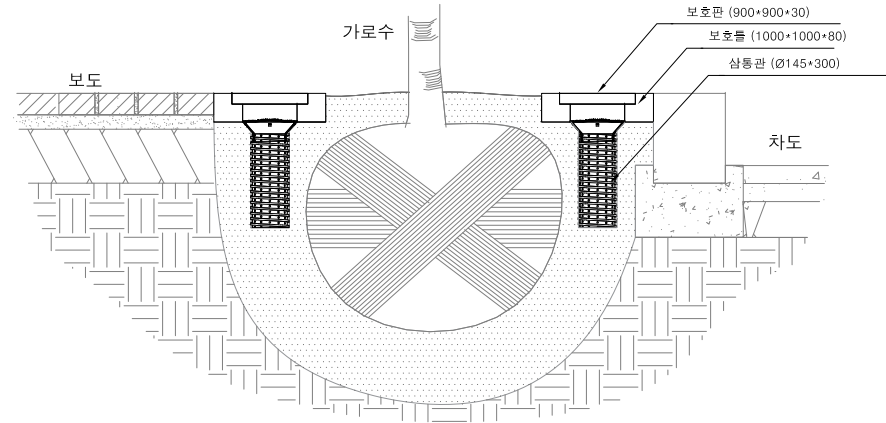
4 보호판 설치단면도 SCALE : NONE
