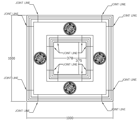
2 보호틀 상세도 SCALE : NONE
