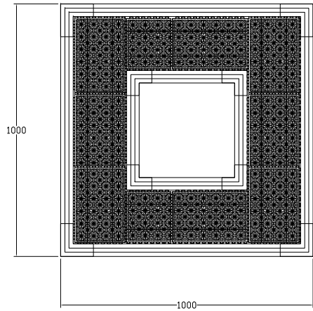
1 가로수보호판 및 보호틀 SCALE : NONE
