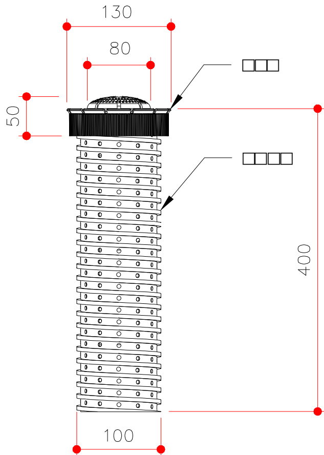
4 생육삼통관 정면도 SCALE = NONE
