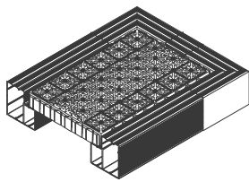
1단 띠녹지보호판 조립도
