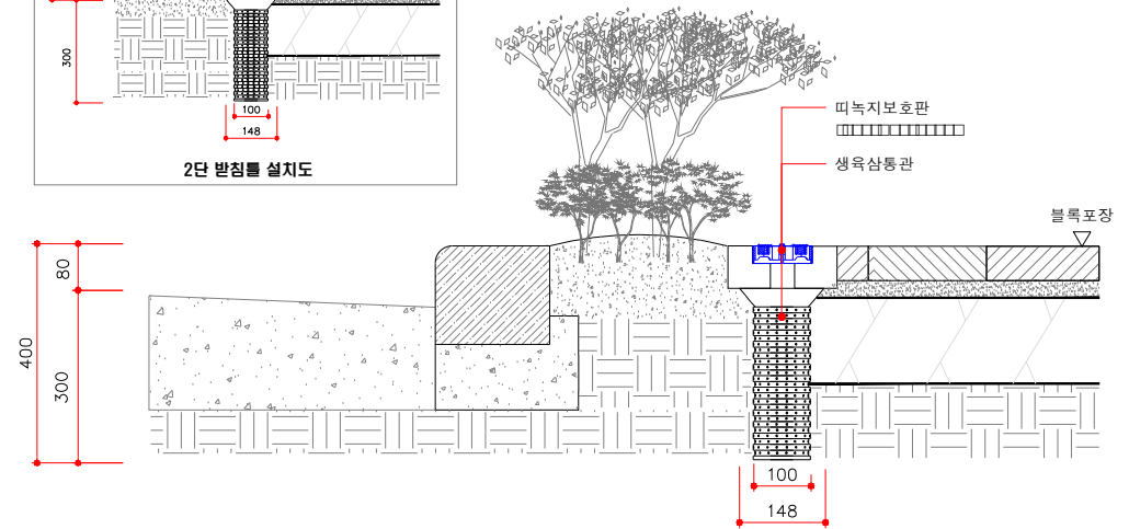
6 1-1' 생육삼통관 결합 설치도 SCALE : NONE
