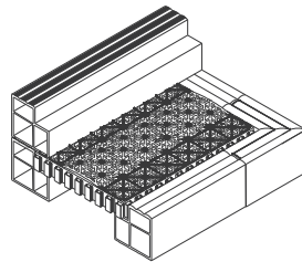
2단 띠녹지보호판 조립도
