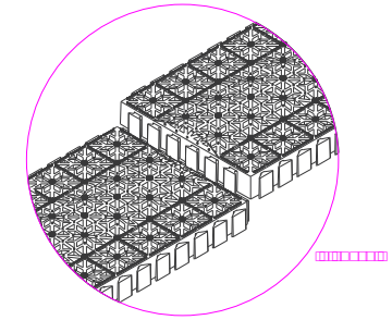
4 보호판 체결 상세도 SCALE = NONE
