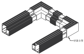
반침틀+연결소켓 조립도
