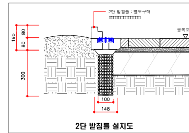
2단 반침틀 설치도
