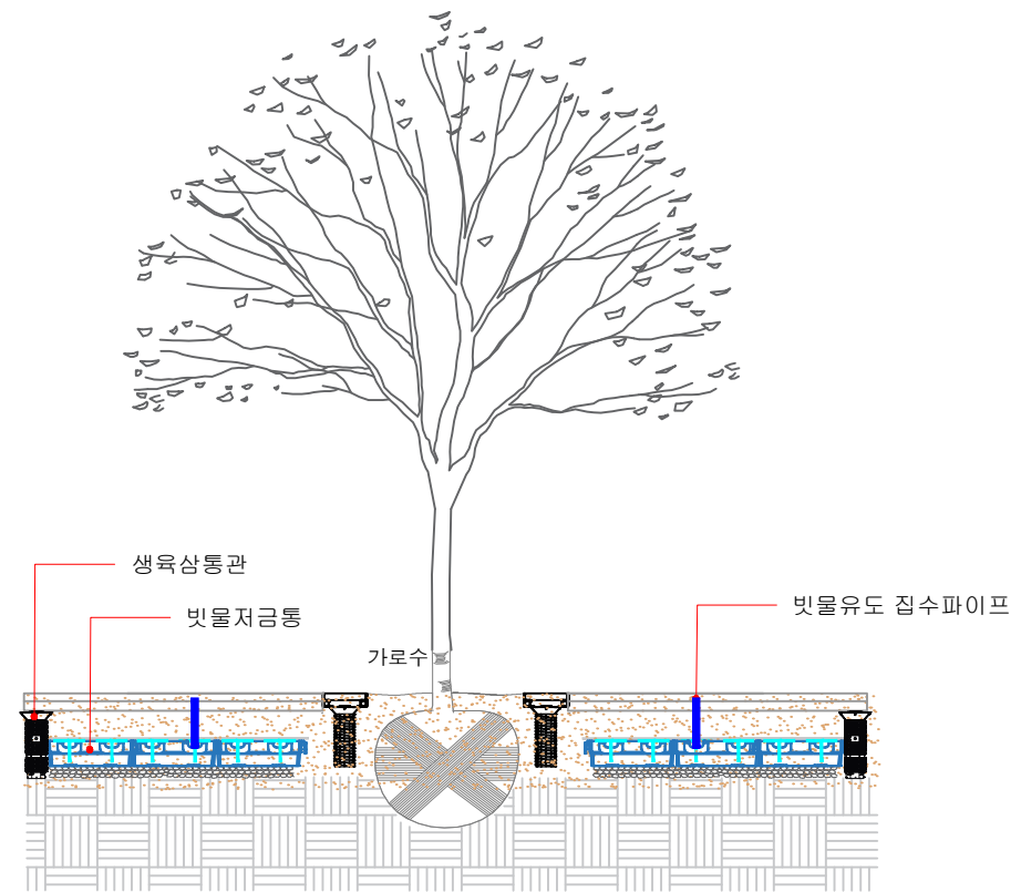
3 B-B' 설치도 SCALE = NONE
