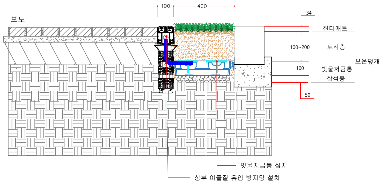
2 A-A' 설치도 SCALE = NONE
