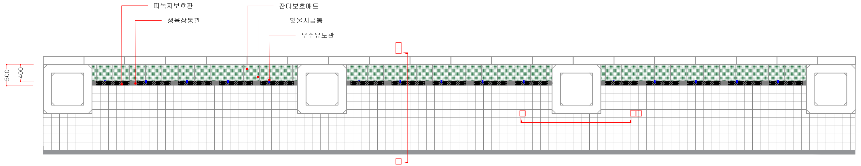
1 생태보행로시스템 평면도 SCALE = NONE
