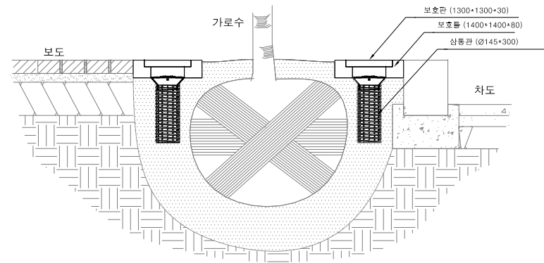
④ 보호판 설치단면도 SCALE : NONE
