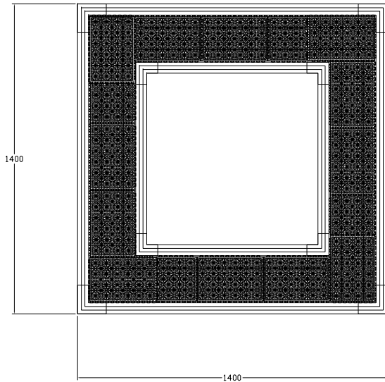
① 가로수보호판 및 보호틀 SCALE : NONE
