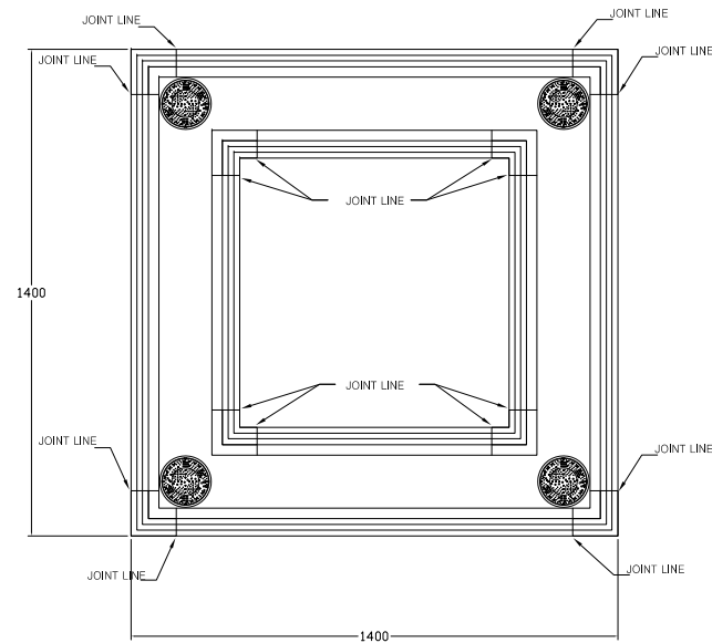
② 보호틀 상세도 SCALE : NONE
