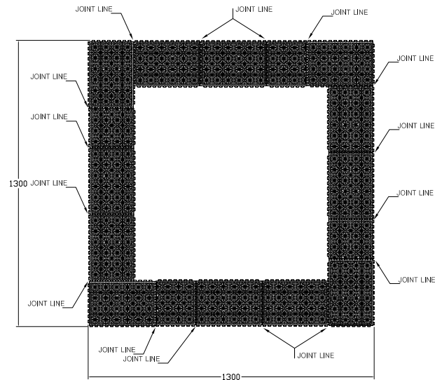
③ 보호판 상세도 SCALE : NONE
