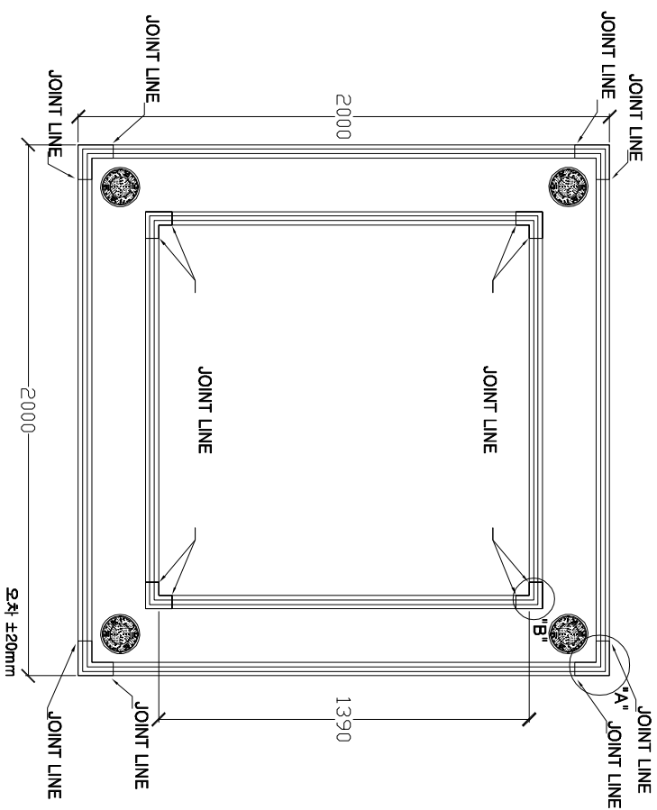
2 보호틀 상세도 SCALE : NONE
