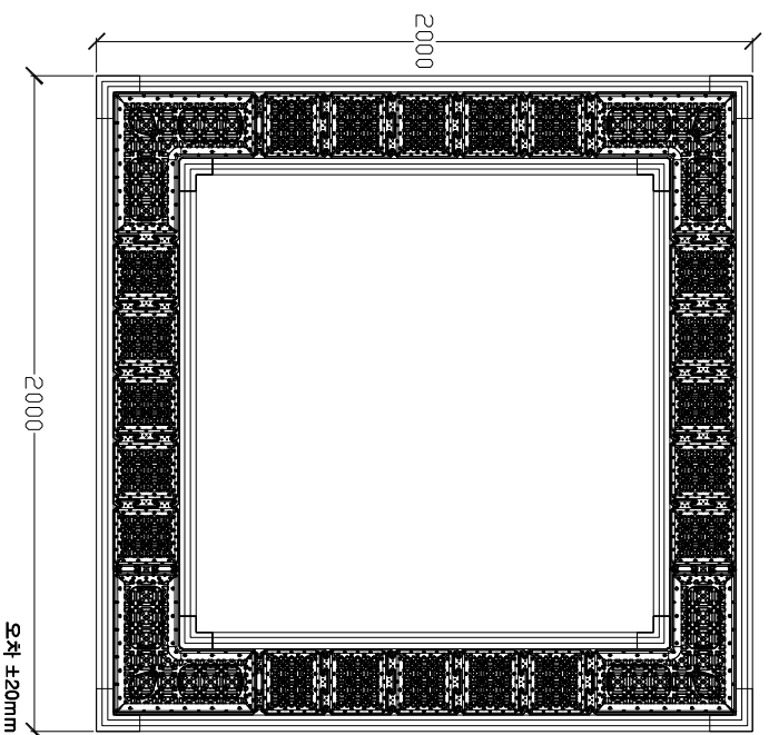
1 가로수보호판 및 보호틀 SCALE : NONE
