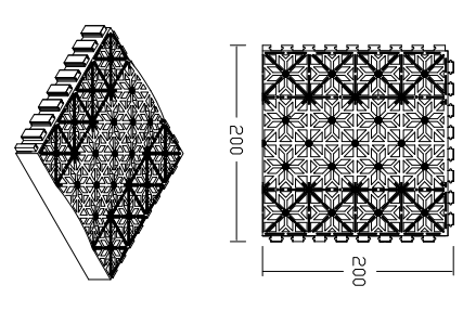
6. 가로수 보호판 B형
