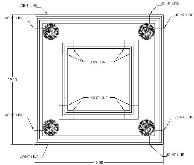
② 보호틀 상세도 SCALE : NONE
