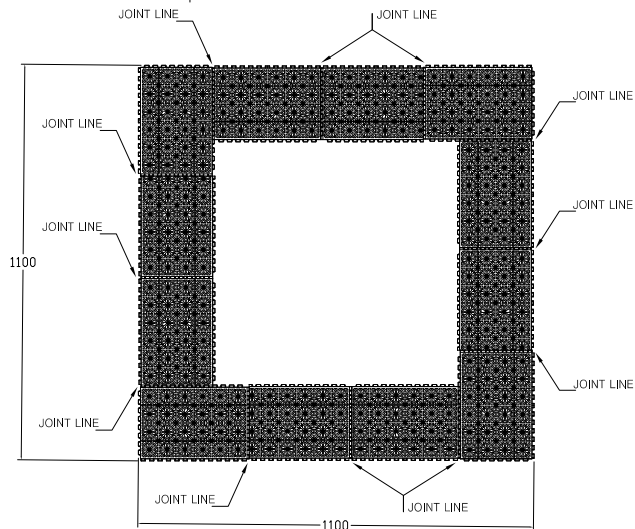
③ 보호판 상세도 SCALE : NONE
