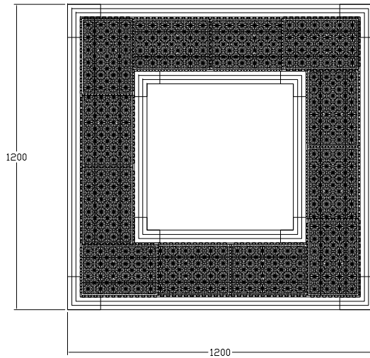
① 가로수보호판 및 보호틀 SCALE : NONE
