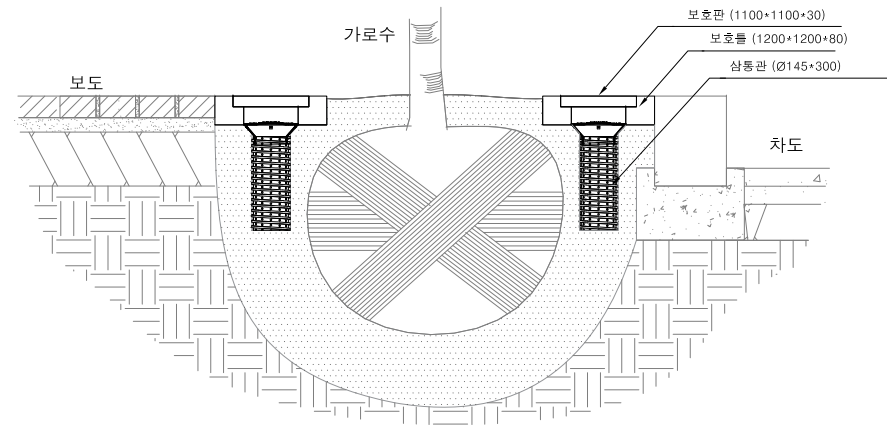
④ 보호판 설치단면도 SCALE : NONE
